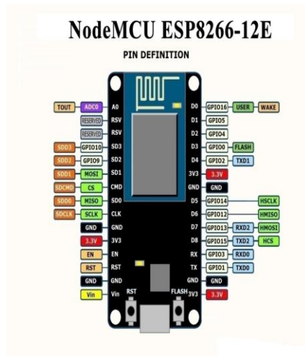
Fig 3. Wi-fi Module ESP8266
